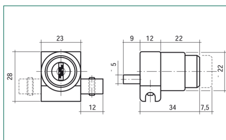
Zár üvegsalathoz
