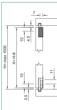
Állítható alsó görgő
