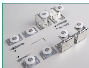
RV30 tolóajtó szett
