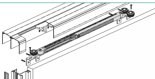
Csillapító szett
