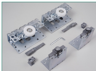
Vasalat szett elől futó ajtóhoz
