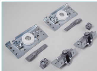
Vasalat szett hátul futó ajtóhoz
