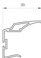
Lider fogantyúprofil
