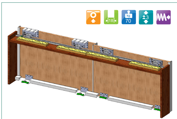
Dupla felső sín porfogó kefével
