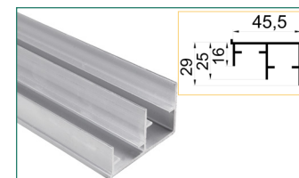
Dupla alsó sín
