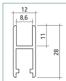
Felső sín
