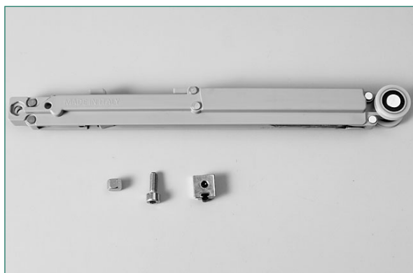
Tolóajtó csillapító 100 Silent, 100 Silent Filo és 100 Silent Glass tolóajtókhoz
