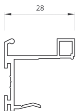
Lider fogantyúprofil
