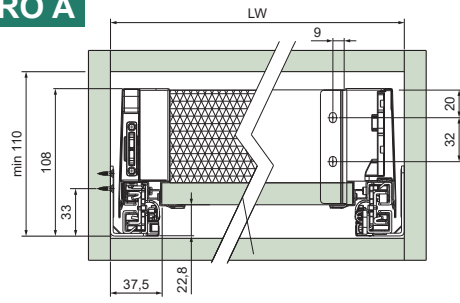
Előlaprögzítő rögzítési pontjai
