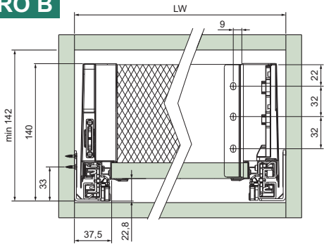
Előlaprögzítő rögzítési pontjai
